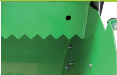
Controcoltello riduce consumi e potenza assorbita Bottom blade decreases fuel consumption
