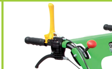
Leve sbloccaggi indipendenti Independent unlocking levers
